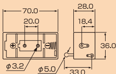
■寸法図 (単位mm)
